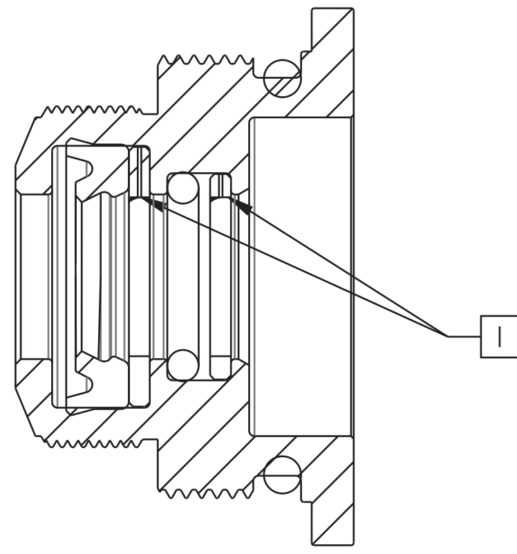
SECTION A-A SCALE 4:1
